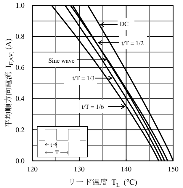
図3 I_{F(AV)} - T_L^{(2)} 特性 ( T_J = 150\text{ }^\circ\text{C} 、 V_R = 200\text{ V} )
