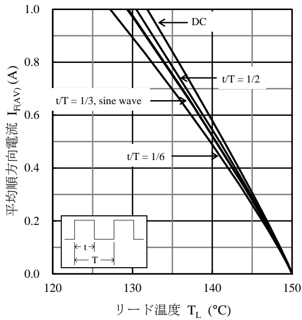
図2 I_{F(AV)} - T_L^{(2)} 特性 ( T_J = 150\text{ }^\circ\text{C} 、 V_R = 0\text{ V} )
