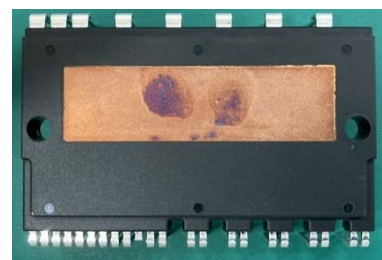
図 4 酸化例 2 (高湿環境保管/製造工程)
