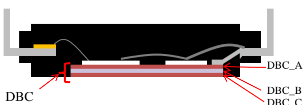
図 1 DBC 構造
