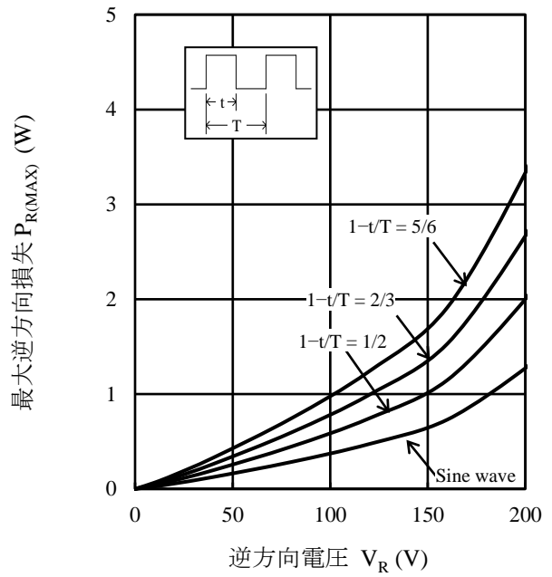
図4 P_{R(MAX)} - V_R 特性 ( T_J = 150^\circ C )
