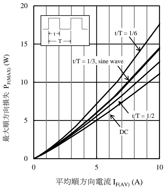
図3 P_{F(MAX)} - I_{F(AV)} 特性 ( T_J = 150^\circ C )
