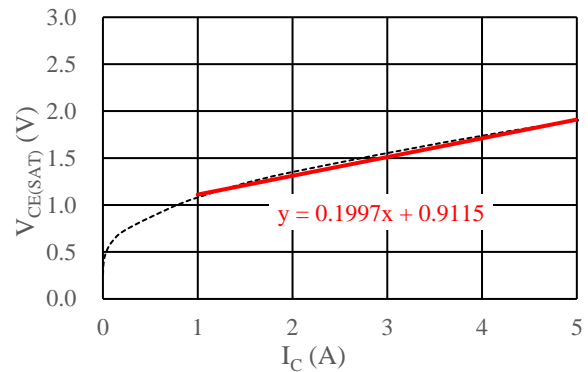
図15-1 V_{CE(SAT)} - I_C 特性の1次近似式
