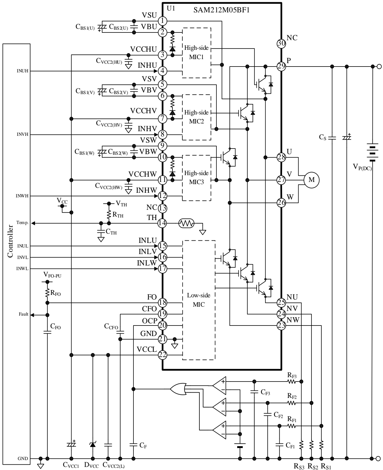
図 10-2 応用回路例 (3 シャント検出方式)
