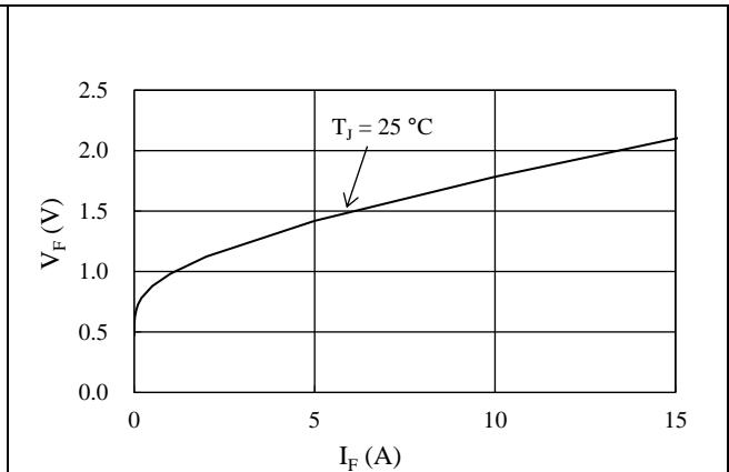
図 16-3 フリーホイールダイオード V_F - I_F 特性
