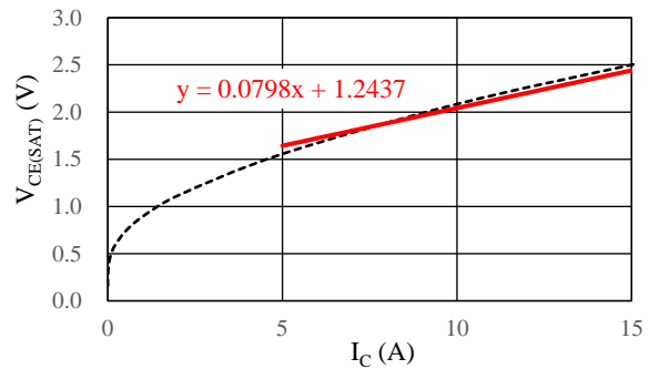
図15-1 V_{CE(SAT)} - I_C 特性の1次近似式
