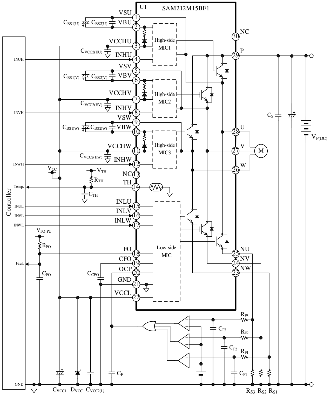
図 10-2 応用回路例 (3 シャント検出方式)
