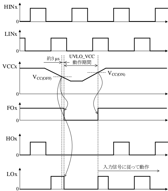
図 12-14 UVLO_VCC 動作波形
