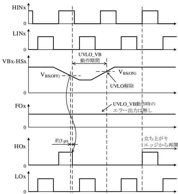
図 12-13 UVLO_VB 動作波形
