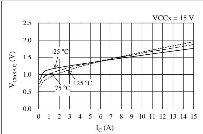
図 15-22 IGBT V_{CE(SAT)} - I_C 特性
