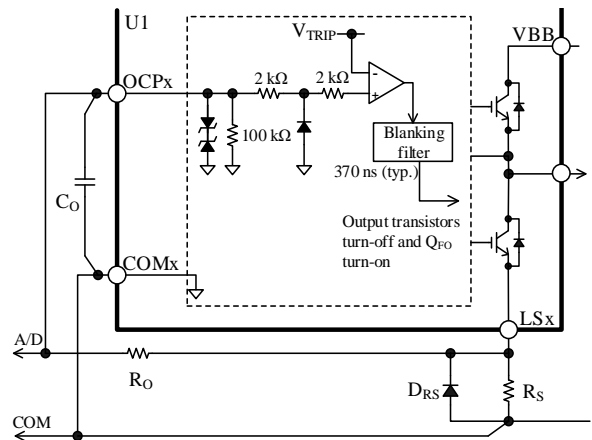
図 12-15 OCPx 端子の周辺回路と内部回路図
