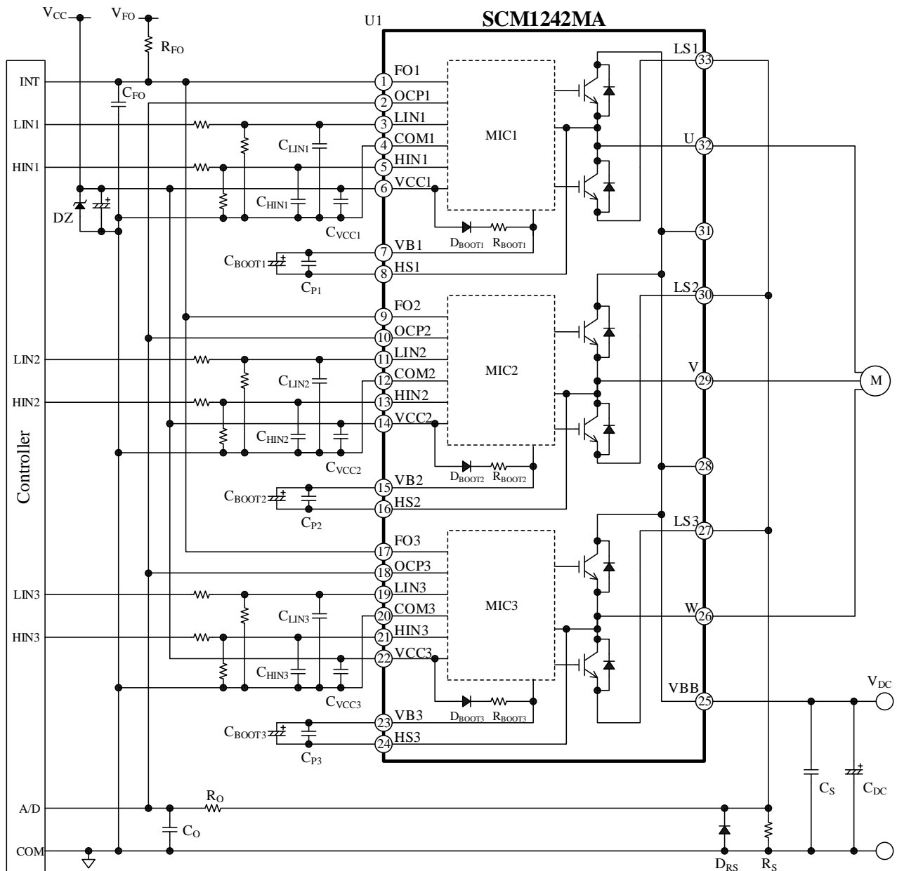
図 9-1 応用回路例 (1 シヤント検出方式)
