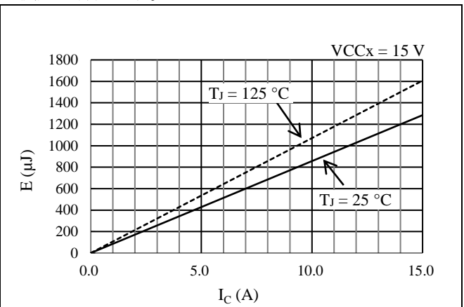
図 15-25 ローサイドスイッチング損失特性
