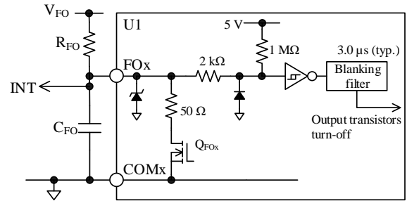
図 12-8 FOx 端子の周辺回路と内部回路
