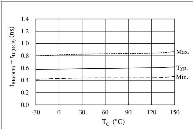
図 15-19 過電流保護ブランキング時間 t_{BK(OCP)} + 内部遅延時間 t_{D(OCP)} 温度特性
