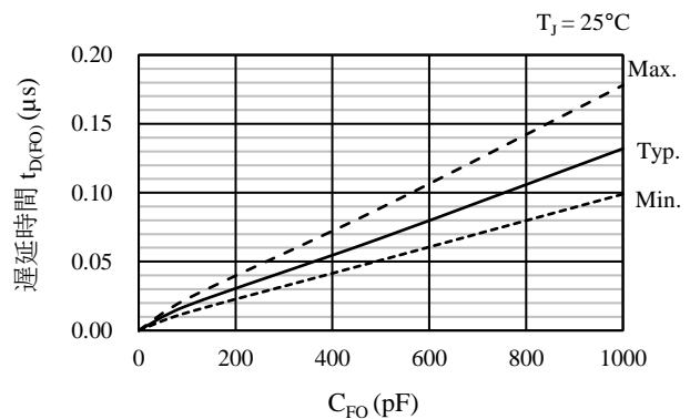
図 12-11 C_{FO} と FOx 端子遅延時間の関係
