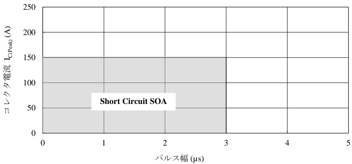
図 15-29 短絡 SOA
