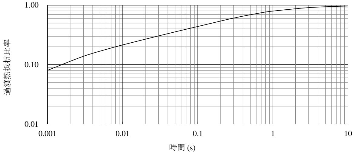
図 15-28 過渡熱抵抗比率
