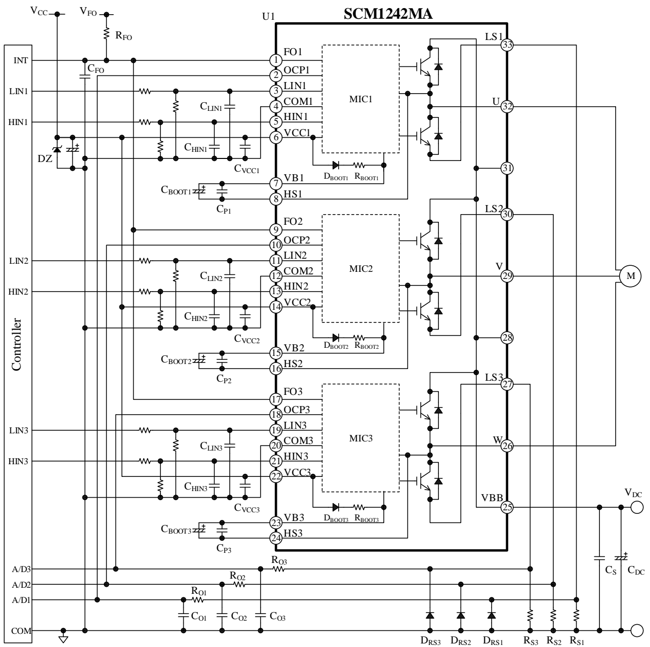
図 9-2 応用回路例 (3 シヤント検出方式)
