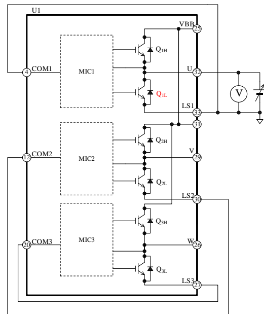
図 13-4 U相ローサイド素子 (Q 1L ) 耐圧測定回路
