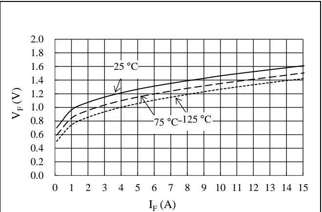
図 15-23 フリーホイールダイオード V_F - I_F 特性
