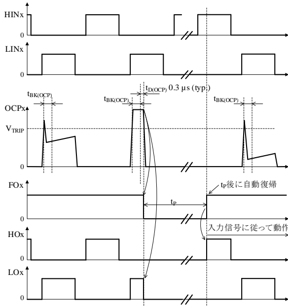
図 12-16 OCP 動作波形
