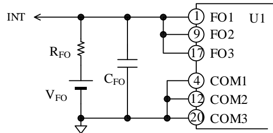
図 12-12 全相シャットダウン回路
