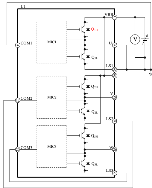
図 13-3 U相ハイサイド素子 (Q 1H ) 耐圧測定回路
