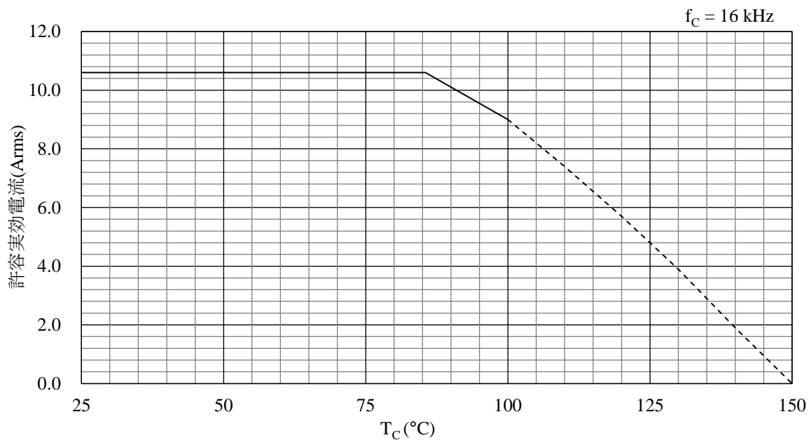
図 15-27 許容電流特性 ( f_c = 16\text{ kHz} )
