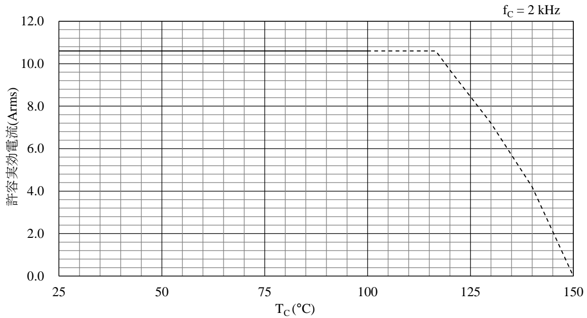
図 15-26 許容電流特性 ( f_c = 2\text{ kHz} )
