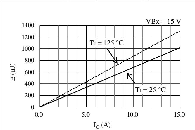
図 15-24 ハイサイドスイッチング損失特性
