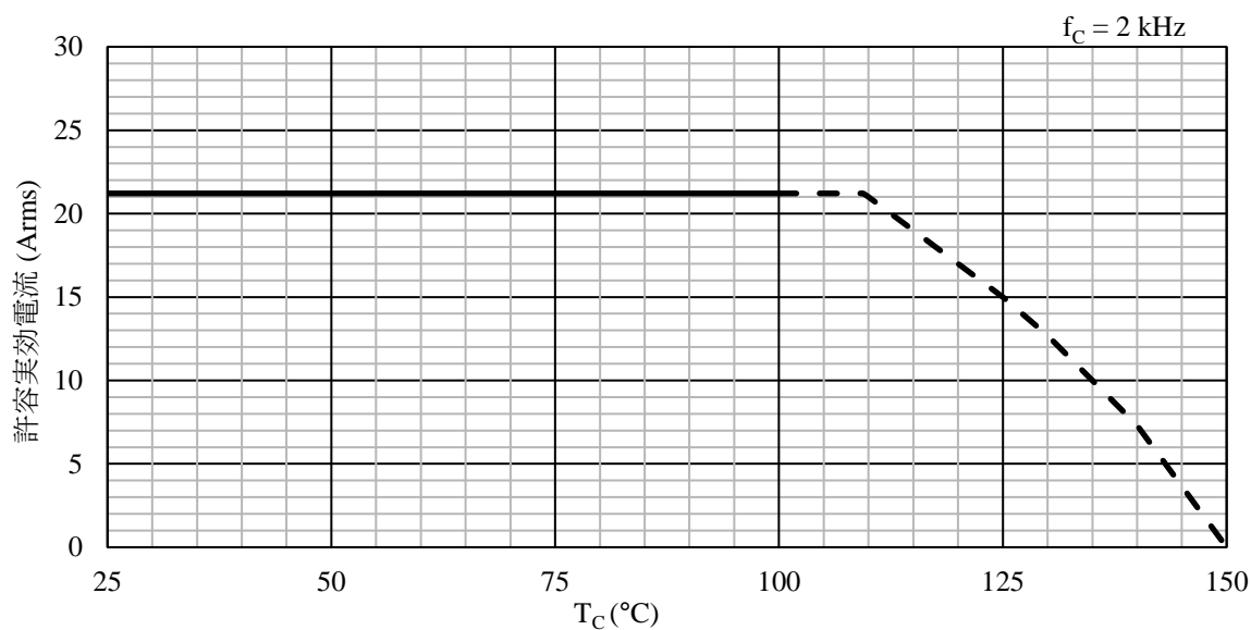
図 15-42 SCM2008MKF 許容電流特性 ( f_c = 2 kHz)
