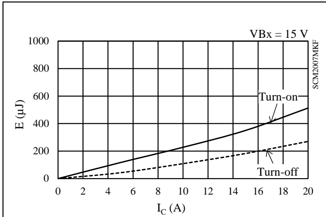
図 15-32 ハイサイドスイッチング損失特性 ( T_J = 25\text{ }^\circ\text{C} )
