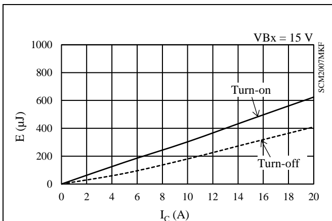
図 15-34 ハイサイドスイッチング損失特性 ( T_J = 125\text{ }^\circ\text{C} )
