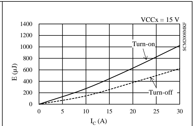
図 15-37 ローサイドスイッチング損失特性 ( T_J = 25\text{ }^\circ\text{C} )
