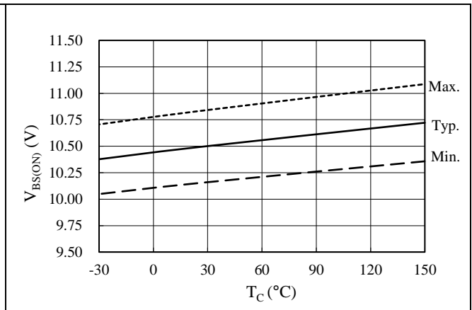
図 15-7 制御動作開始電圧 V_{BS(ON)} 温度特性
