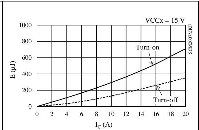
図 15-33 ローサイドスイッチング損失特性 ( T_J = 25\text{ }^\circ\text{C} )
