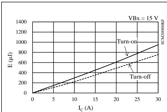
図 15-38 ハイサイドスイッチング損失特性 ( T_J = 125\text{ }^\circ\text{C} )
