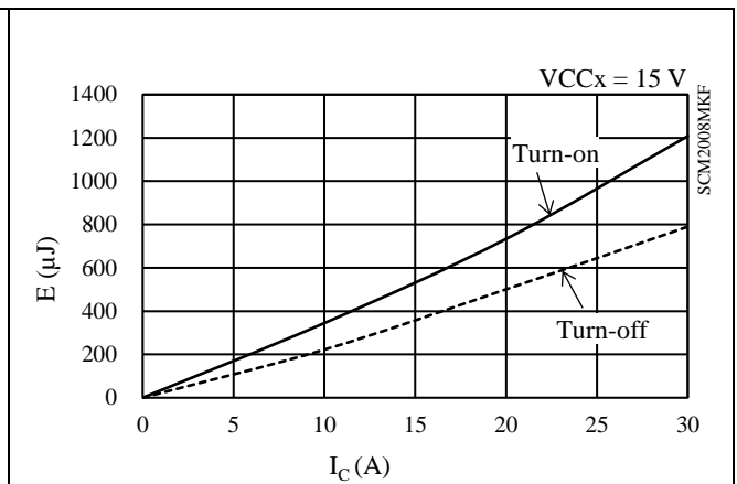
図 15-39 ローサイドスイッチング損失特性 ( T_J = 125\text{ }^\circ\text{C} )
