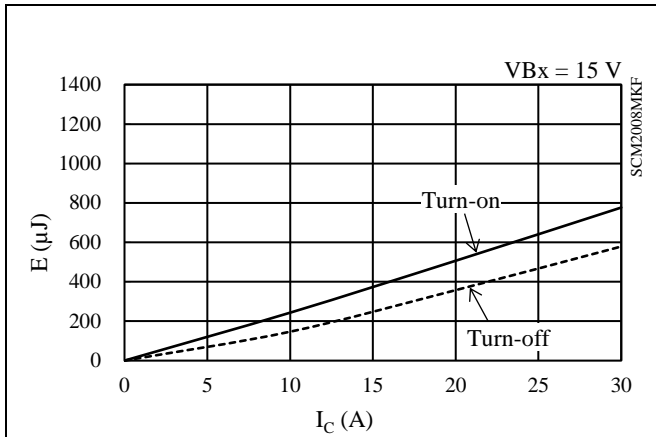
図 15-36 ハイサイドスイッチング損失特性 ( T_J = 25\text{ }^\circ\text{C} )
