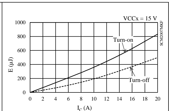
図 15-35 ローサイドスイッチング損失特性 ( T_J = 125\text{ }^\circ\text{C} )
