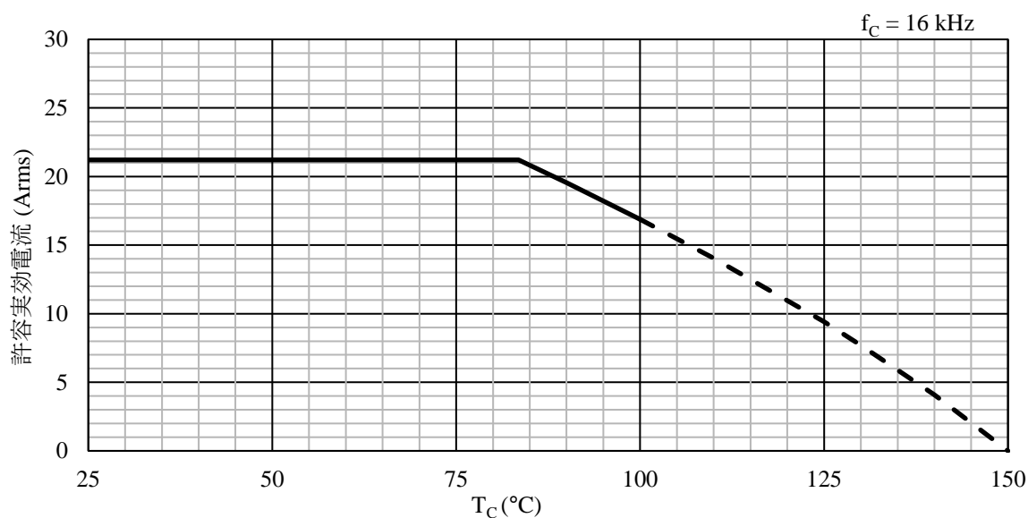
図 15-43 SCM2008MKF 許容電流特性 ( f_c = 16 kHz)
