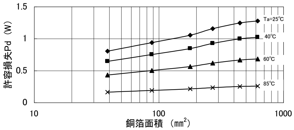
銅箔面積—許容損失 T_{jmax}=100^{\circ}C
