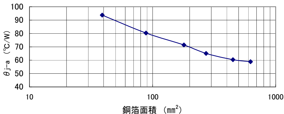
SI-8000TMX 銅箔面積—熱抵抗
