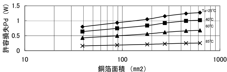
銅箔面積—許容損失 T jmax =100°C
