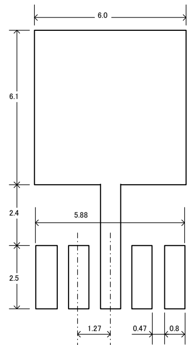
ソルダーパターン設計例
