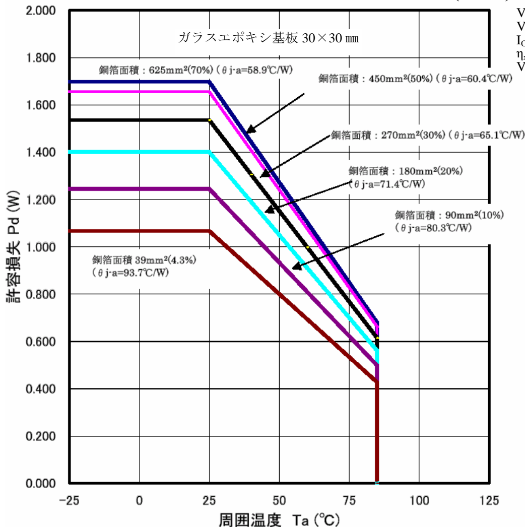
SI-8000TM シリーズ熱減定格曲線
