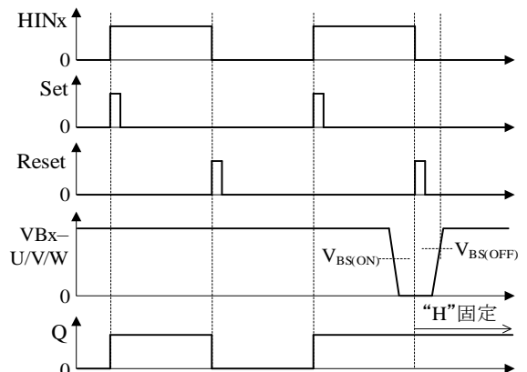
図 12-3 VB_x-U/V/W 間電圧低下による誤動作波形
