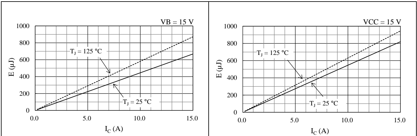
図 15-23 ハイサイドスイッチング損失特性
