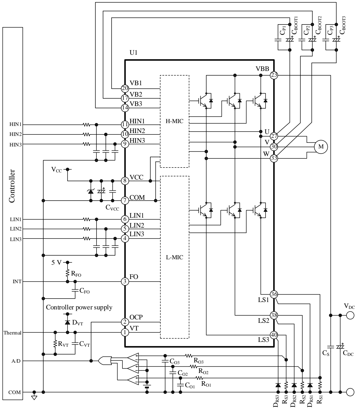
図 9-2 応用回路例 (3チャンネル検出方式)
