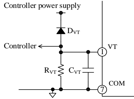
図 12-12 VT 端子周辺回路
