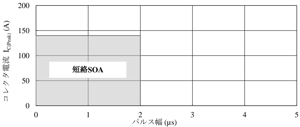
図 15-28 短絡 SOA
