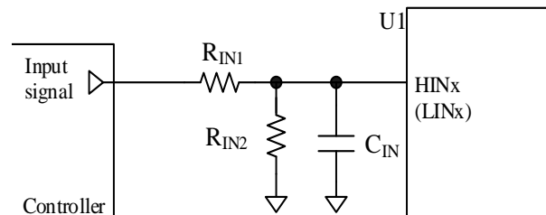
図 12-6 HIN x 端子、LIN x 端子のフィルタ回路
