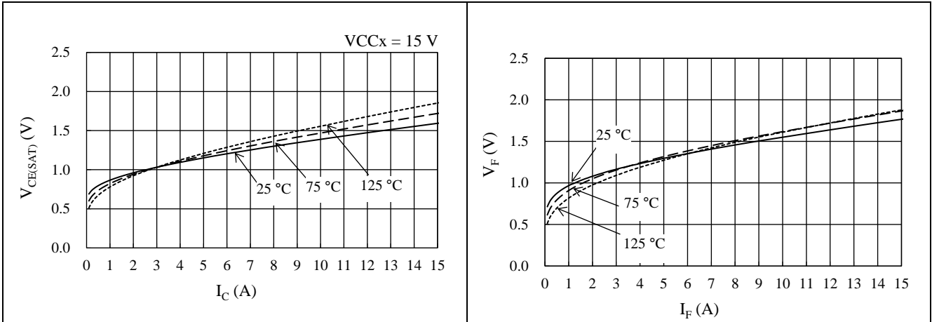
図 15-21 IGBT V_{CE(SAT)} - I_C 特性
