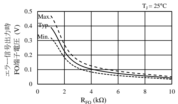
図 12-10 エラー信号出力時 FO 端子電圧 - プルアップ抵抗 R_{FO} 特性
