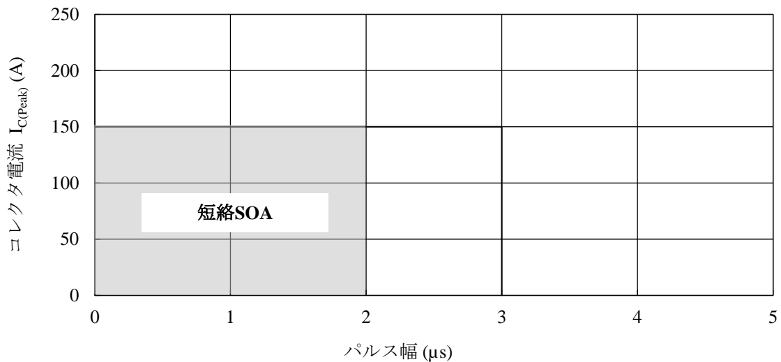
図 15-28 短絡 SOA
