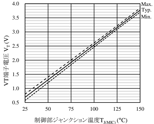
図 12-13 VT 端子電圧 V T 温度特性（設計値）
