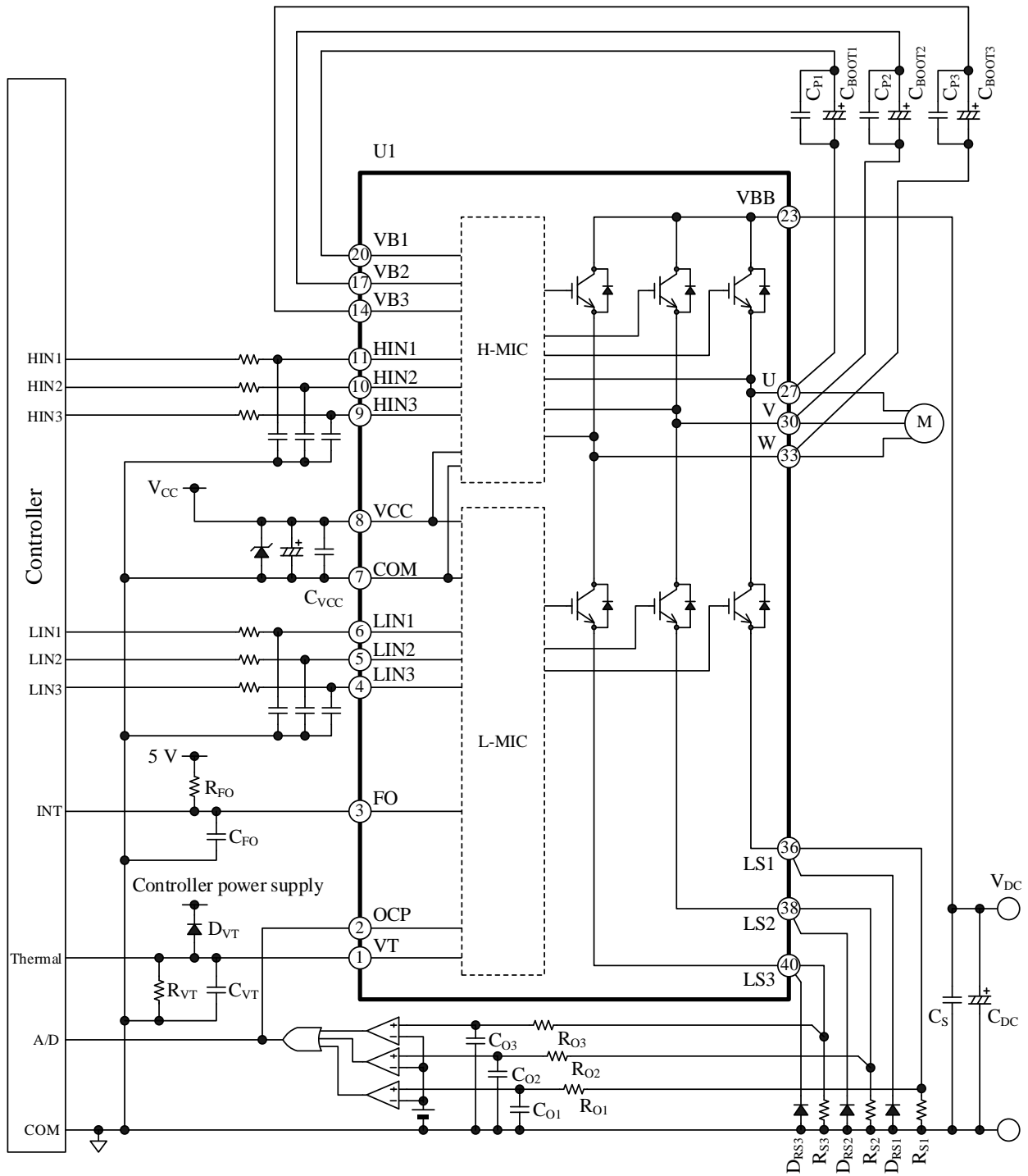
図 9-2 応用回路例 (3 シヤント検出方式)
