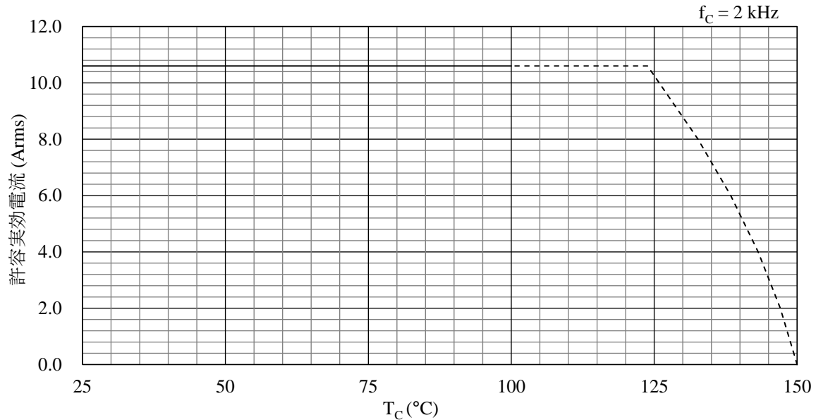
図 15-25 許容電流特性 ( f_c = 2 \text{ kHz} )
