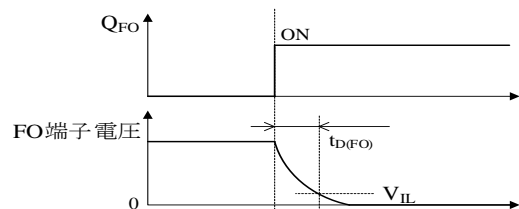
図 12-9 FO 端子の遅延時間 t_{D(FO)}
