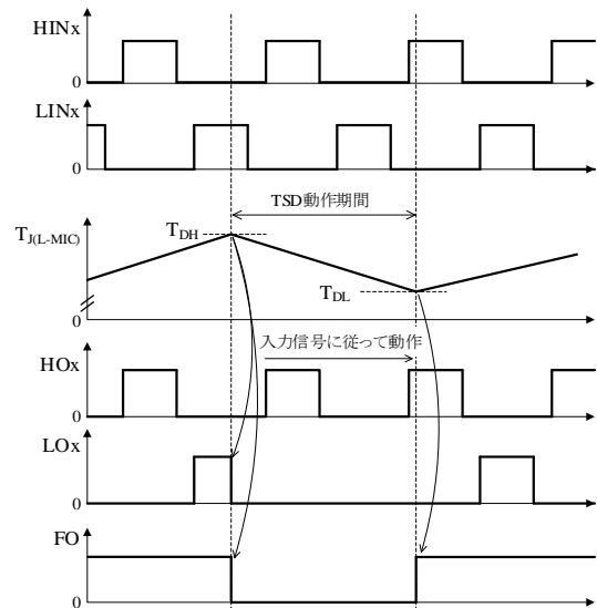
図 12-18 TSD 動作波形
