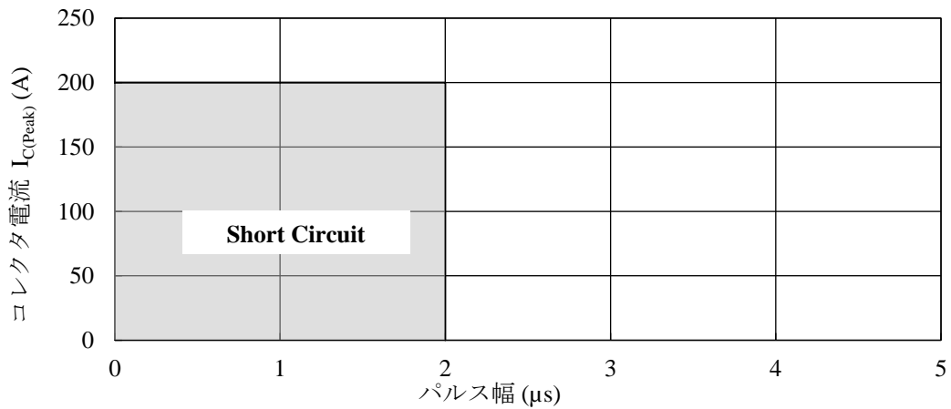
図 15-28 短絡 SOA
