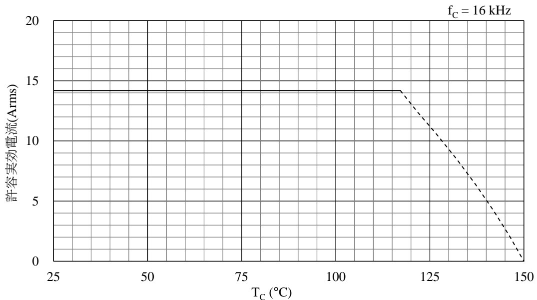
図 15-26 許容電流特性 ( f_c = 16 kHz)
