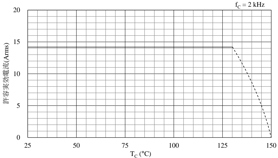
図 15-25 許容電流特性 ( f_c = 2 kHz)
