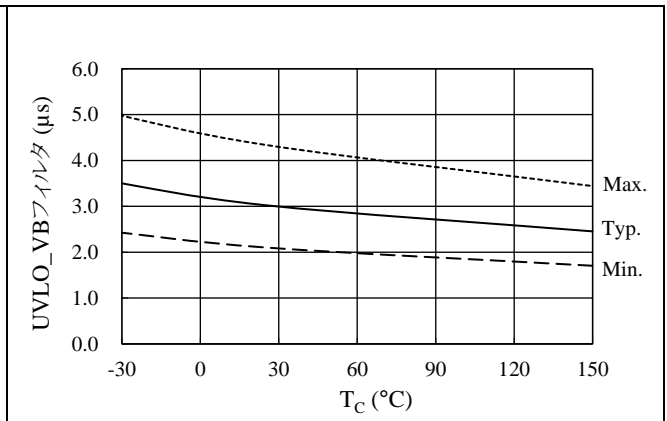
図 15-10 UVLO_VB フィルタ時間温度特性
