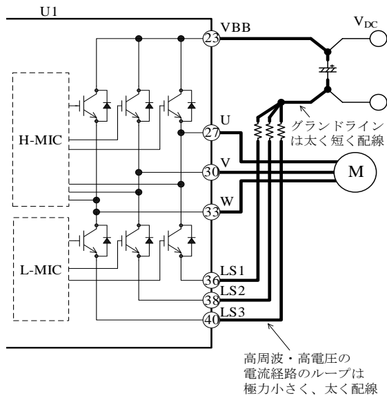
図 13-1 高周波かつ高電圧の電流経路
