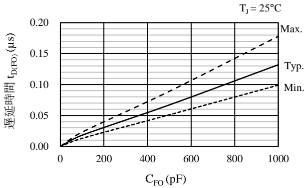
図 12-11 C FO と FO 端子遅延時間の関係
