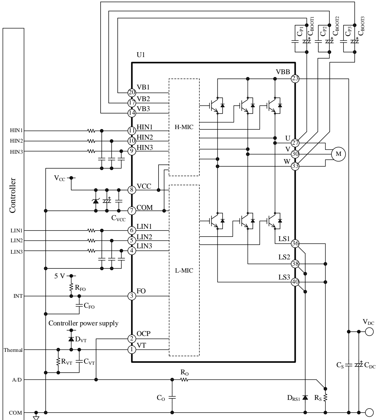
図 9-1 応用回路例 (1 シャフト検出方式)
