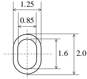
1ピン～20ピン
