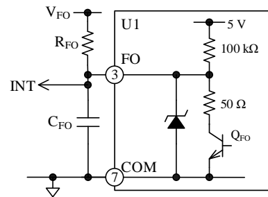
図 12-8 FO 端子の周辺回路と内部回路
