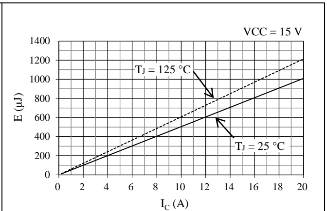
図 15-4 ローサイドスイッチング損失特性
