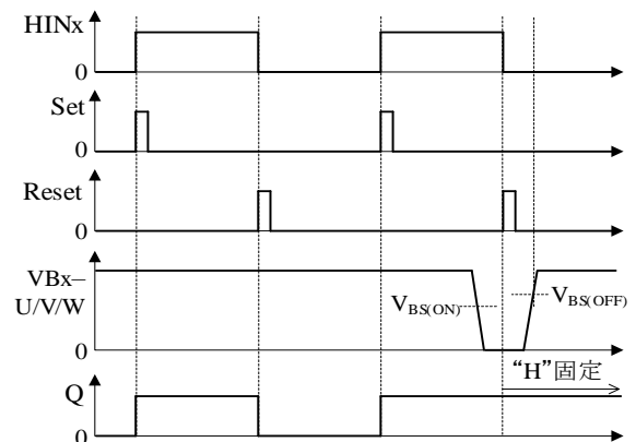
図 12-3 VB_x-U/V/W 間電圧低下による誤動作波形
