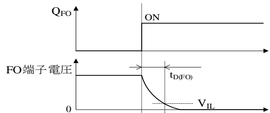
図 12-9 FO 端子の遅延時間 t_{D(FO)}
