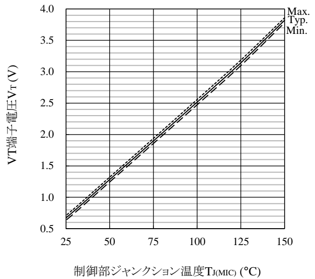
図 12-13 VT 端子電圧 V T 温度特性（設計値）
