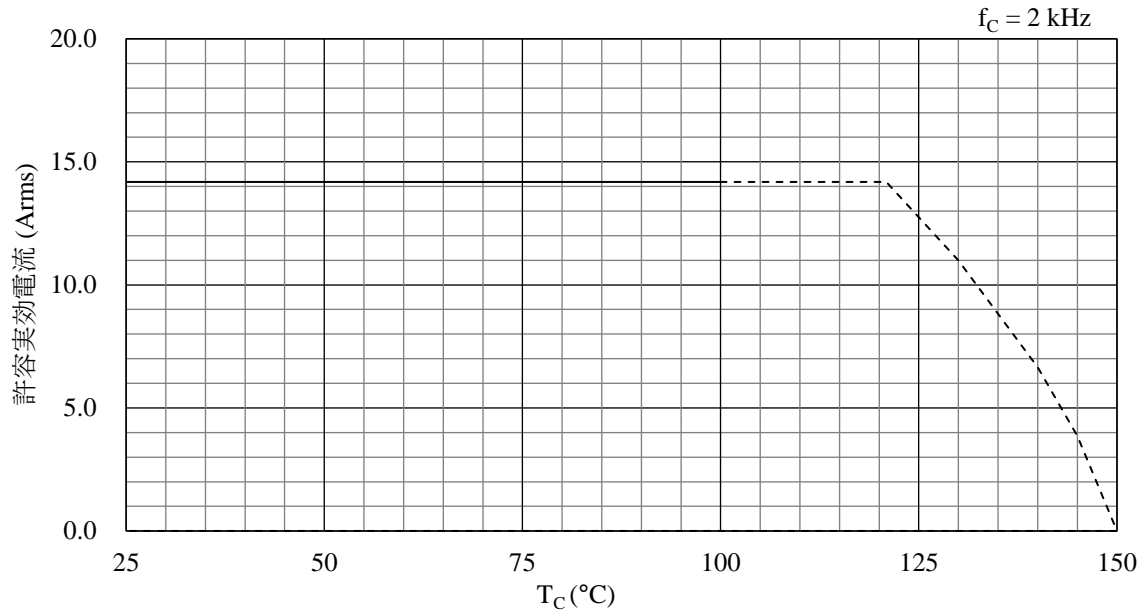
図 15-5 許容電流特性 ( f_c = 2 \text{ kHz} )
