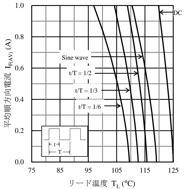
図3 I_{F(AV)} - T_L 代表特性 ( T_J = 125\text{ }^\circ\text{C} 、 V_R = 15\text{ V} )
