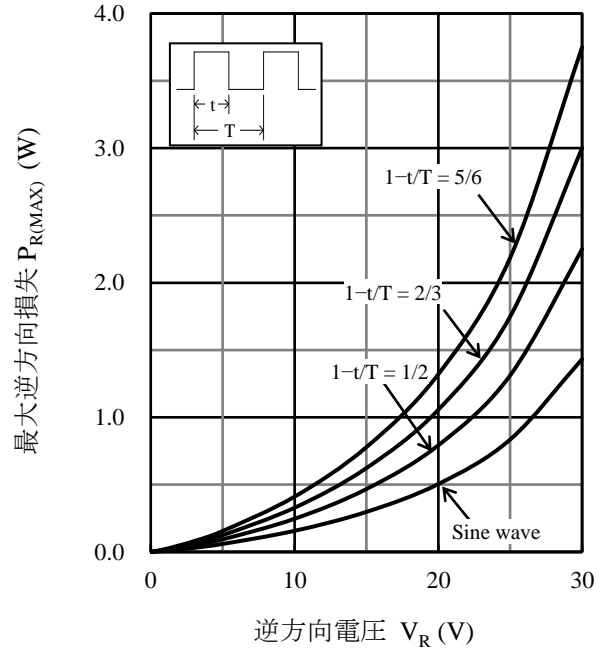
図6 P_{R(MAX)} - V_R 特性 ( T_J = 125\text{ }^\circ\text{C} )
