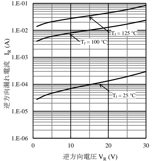
図8 I_R - V_R 代表特性
