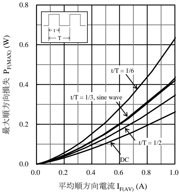
図5 P_{F(MAX)} - I_{F(AV)} 特性 ( T_J = 125\text{ }^\circ\text{C} )
