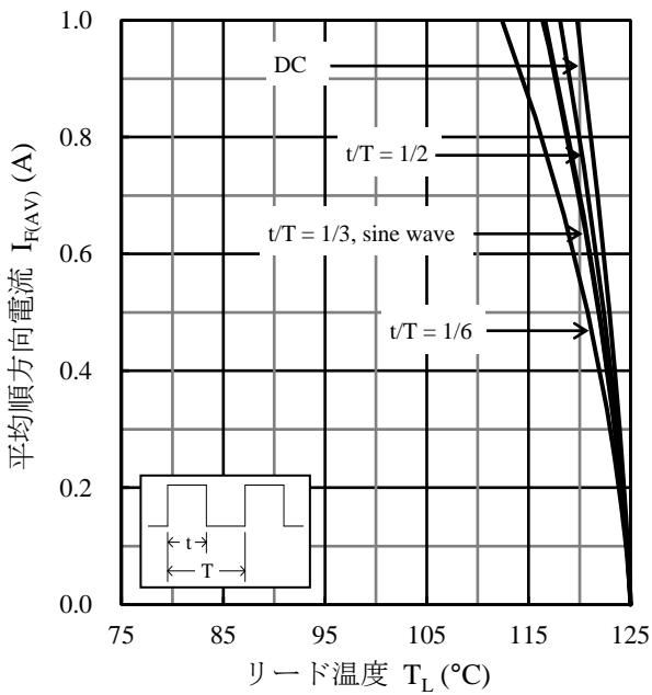
図2 I_{F(AV)} - T_L 特性 ( T_J = 125\text{ }^\circ\text{C} 、 V_R = 0\text{ V} )
