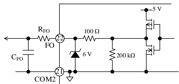
図 11-11 FO 端子の周辺回路と内部回路
