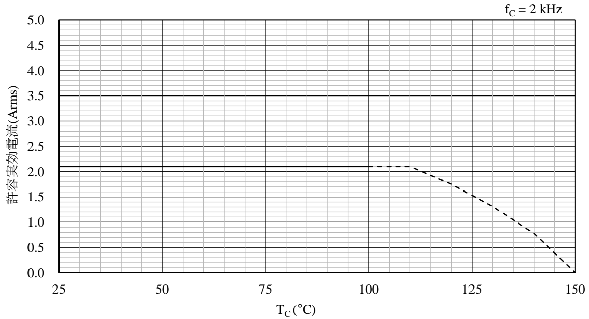
図 14-29 許容電流特性 ( f_C = 2\text{ kHz} )
