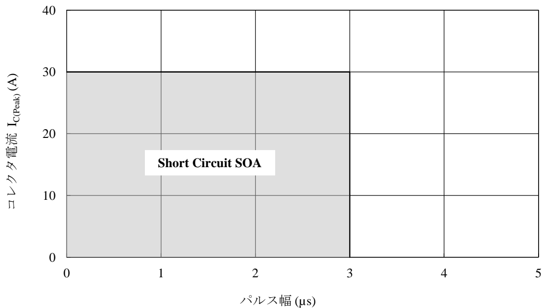
図 14-31 短絡 SOA
