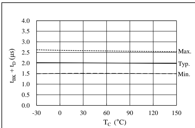
図 14-24 過電流保護ブランキング時間 t_{BK} + 内部遅延時間 t_D 温度特性
