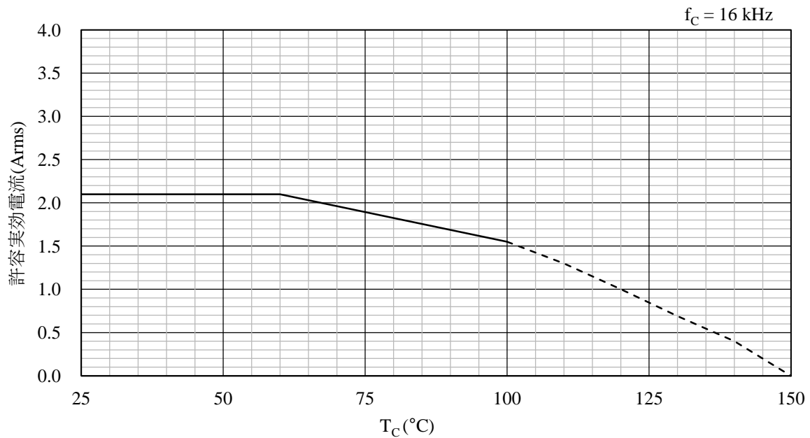
図 14-30 許容電流特性 ( f_C = 16\text{ kHz} )
