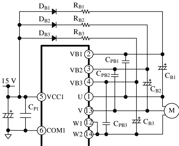
図 11-2 ブートストラップ回路
