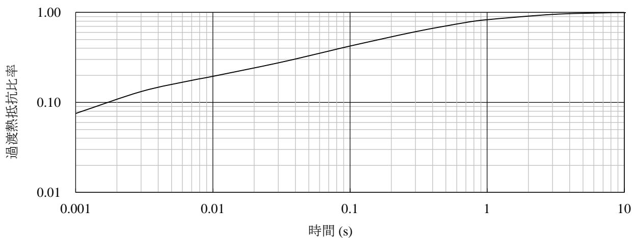
図 14-1 SLA6805MH 過渡熱抵抗比率
