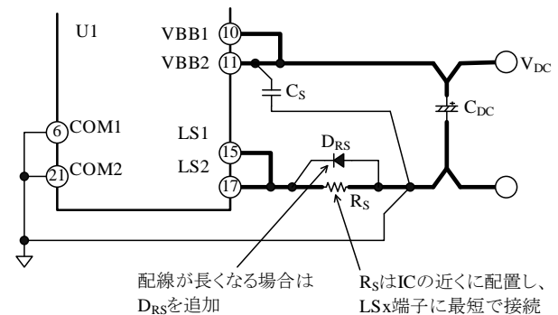
図 11-1 LSx 端子周りの配線
