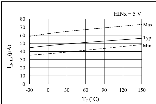
図 14-16 HINx 端子入力電流 I_{IN(H)} 温度特性
