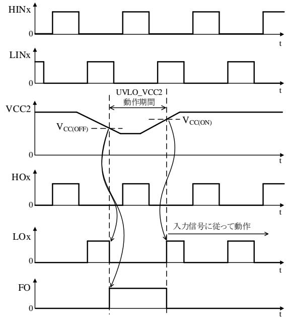
図 11-14 UVLO_VCC2 動作波形
