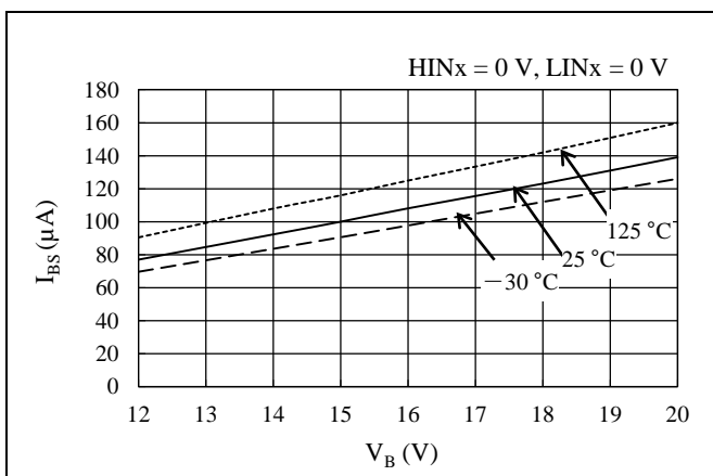
図 14-6 V_{Bx} 端子電圧 V_B - 制御電源電流 I_{BS} 特性 ( HIN_x = 0 V )
