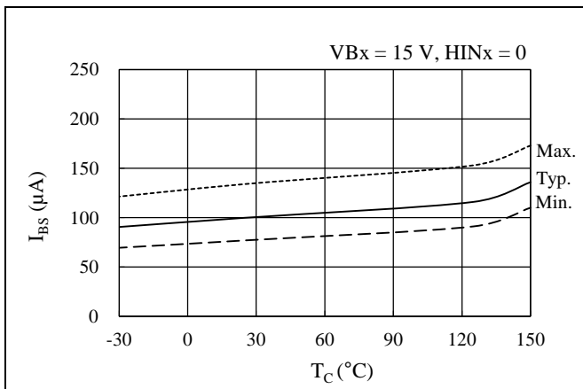
図 14-4 制御電源電流 (1 相) I_{BS} 温度特性 ( HIN_x = 0 V )
