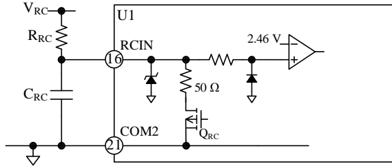
図 11-9 RCIN 端子の周辺回路と内部回路
