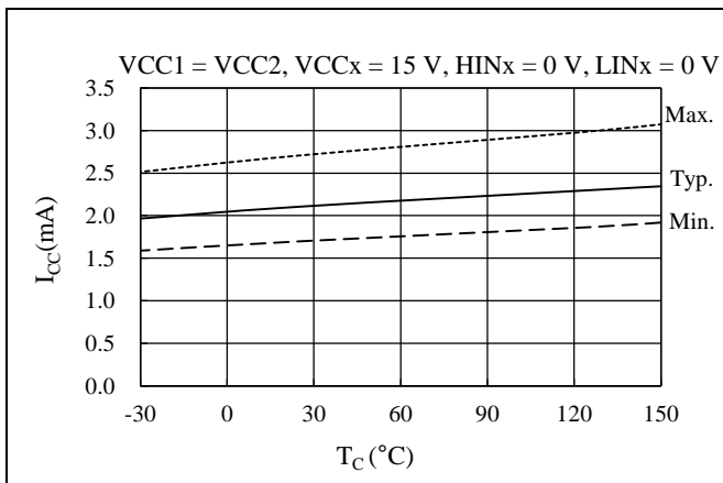
図 14-2 制御電源電流 I_{CC} 温度特性 ( HIN_x = 0 V 、 LIN_x = 0 V )
