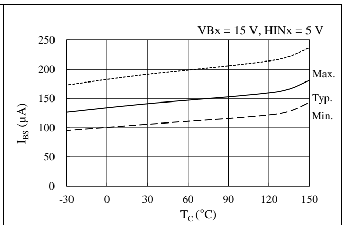
図 14-5 制御電源電流 (1 相) I_{BS} 温度特性 ( HIN_x = 5 V )
