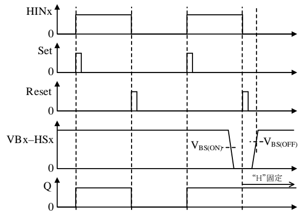
図 11-4 \text{VBx} 端子と出力端子間の電圧低下による誤動作波形
