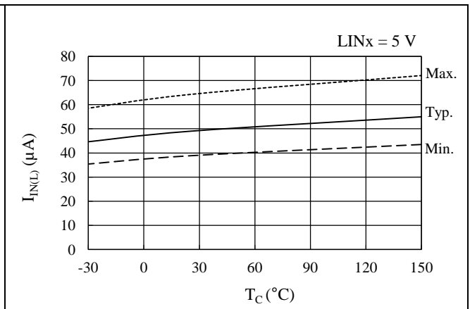
図 14-17 LINx 端子入力電流 I_{IN(L)} 温度特性
