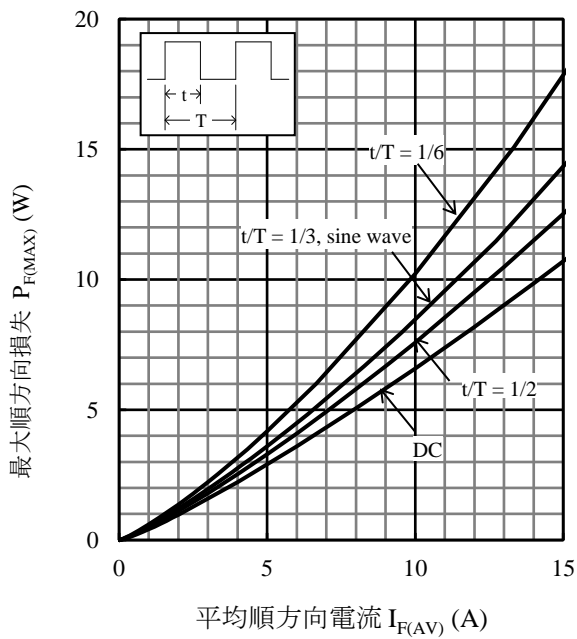
図5 P_{F(MAX)} - I_{F(AV)} 特性 ( T_J = 150\text{ }^\circ\text{C} )
