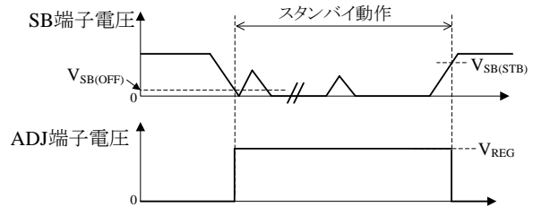
図 8-23 PFC ON/OFF 機能
