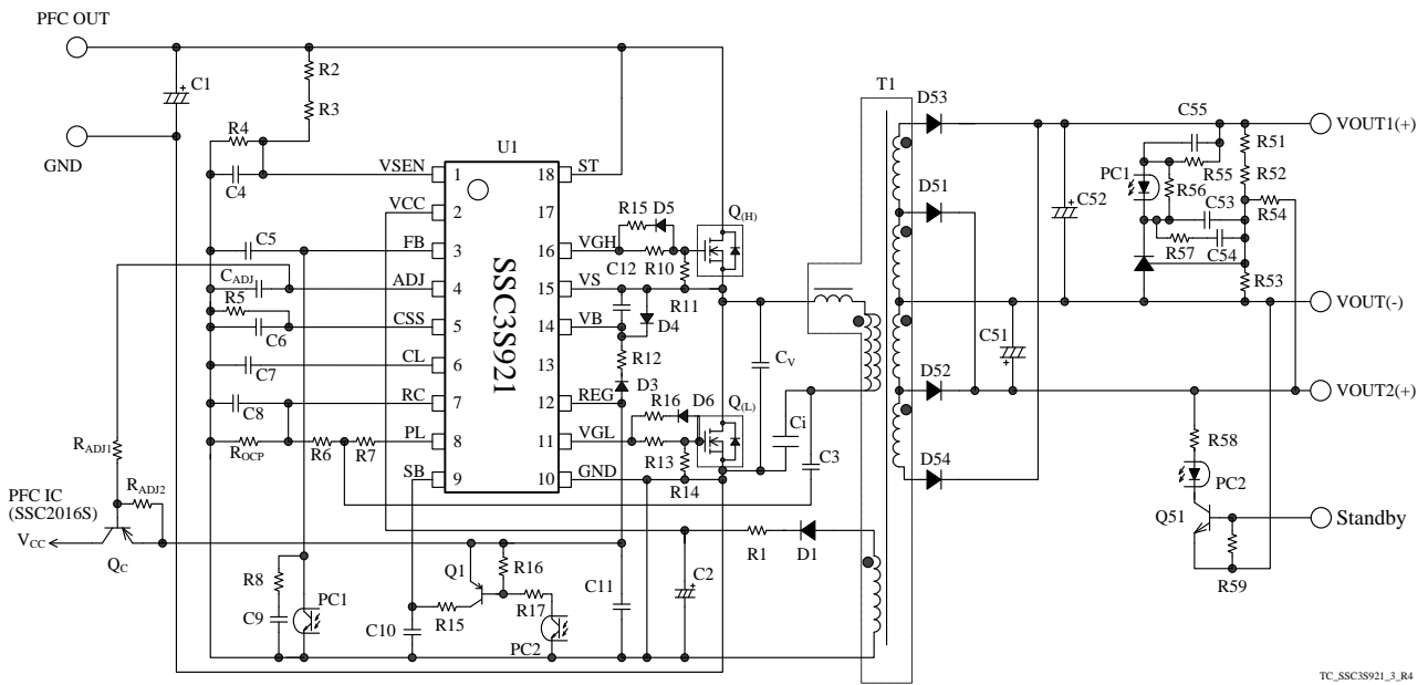
図 5-1 応用回路例
