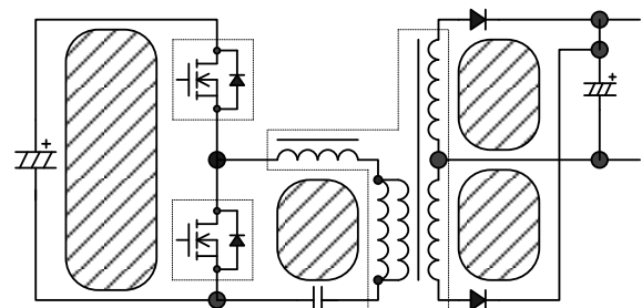
図 9-3 高周波電流ループ
