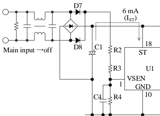
図 8-33 入力コンデンサの残留電圧放電
