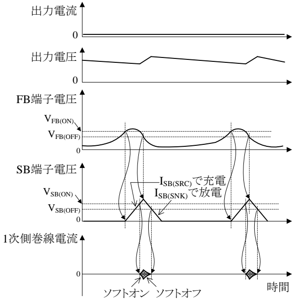
図 8-22 バースト発振動作
