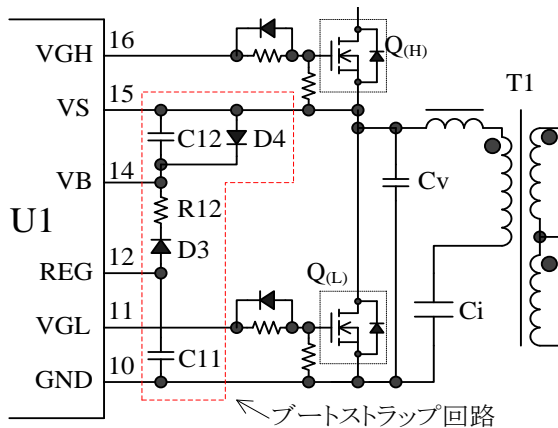
図 8-17 ブートストラップ回路
