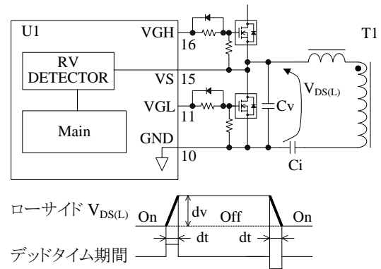
図 8-24 VS 端子とデッドタイム期間
