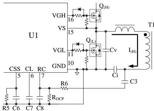
図 8-38 RC 端子周辺回路
