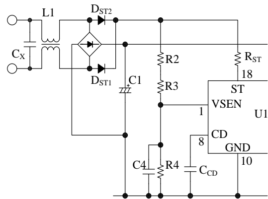
図 8-36 VSEN 端子周辺回路
