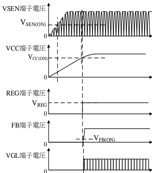
図 8-12 起動動作波形
