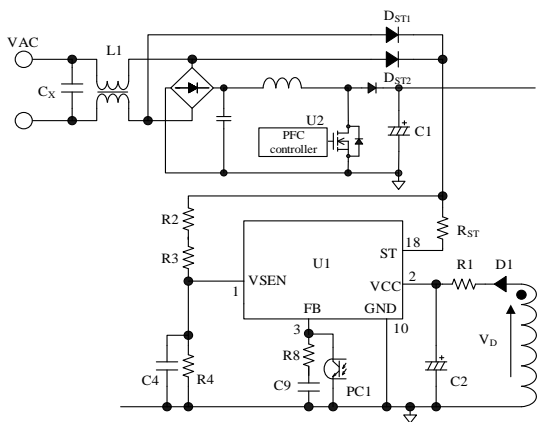
図 8-11 VCC 端子周辺回路
