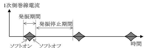
図 8-19 スタンバイ動作波形
