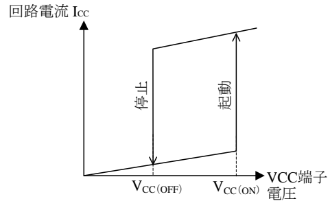
図 8-13 VCC 端子電圧と回路電流 I_{CC}
