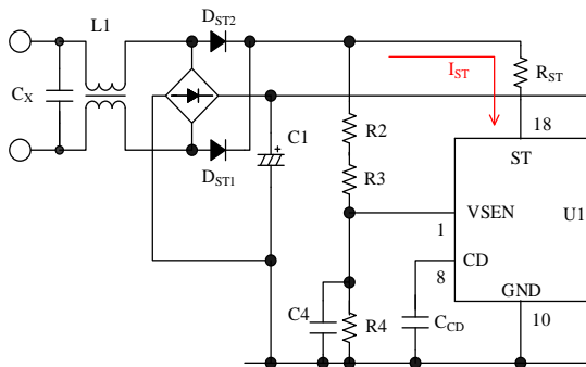
図 8-31 ST 端子周辺回路
