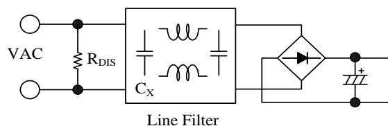
図 8-30 入力部ラインフィルタ標準回路
