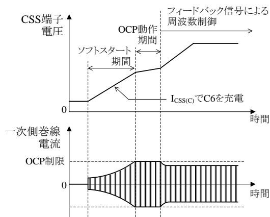
図 8-15 ソフトスタート動作
