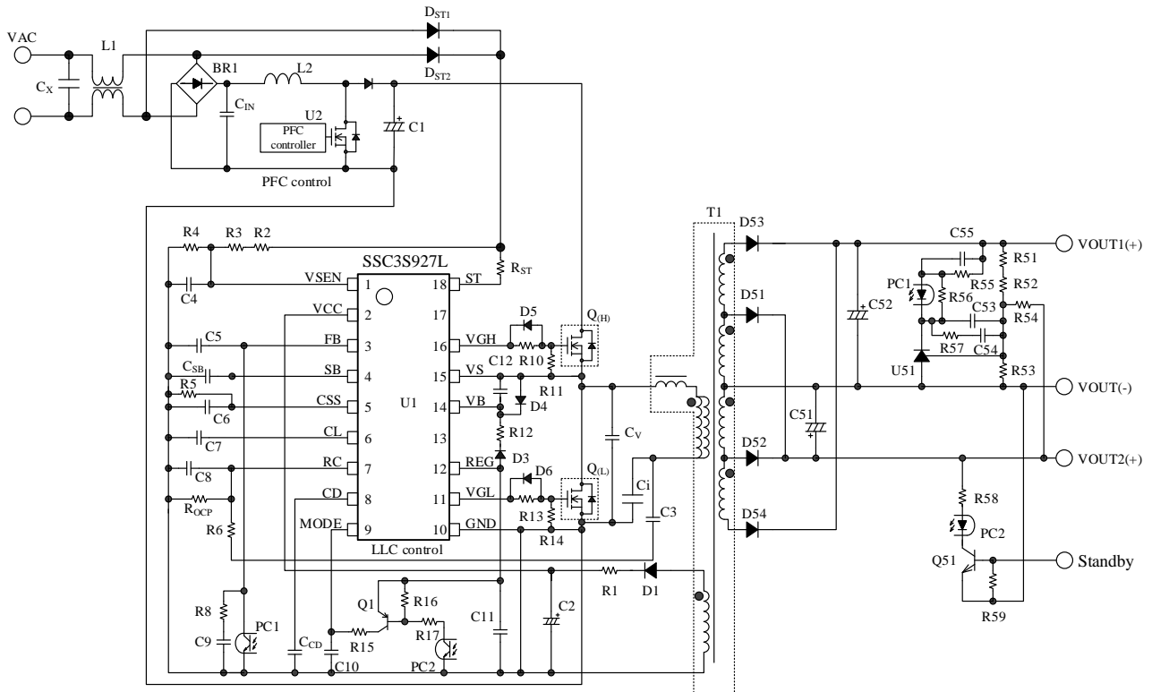
図 5-1 応用回路例
