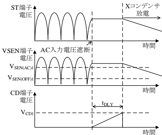
図 8-32 X コンデンサ放電機能動作波形
