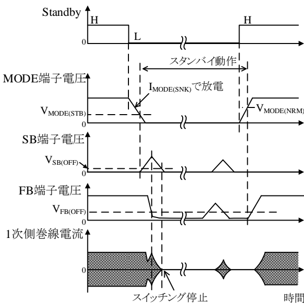
図 8-21 スタンバイ切り替え動作波形
