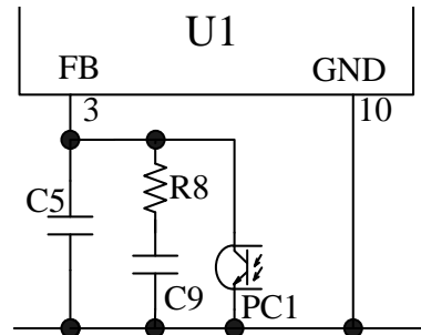
図 8-18 FB 端子周辺回路
