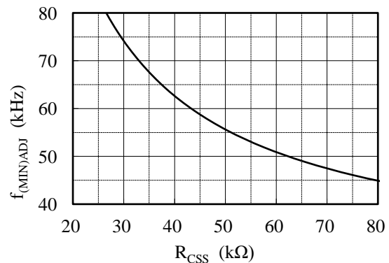
図 8-16 R5 ( R_{CSS} ) と f_{(MIN)ADJ} 特性
