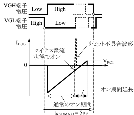
図 8-33 ハイサイドオン期間のリセット検出機能動作例
