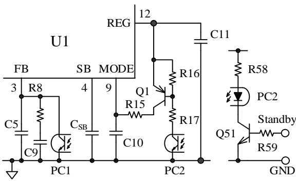
図 8-20 スタンバイ切り替え回路
