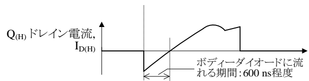
図 8-25 ZCS 確認箇所
