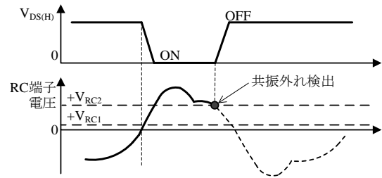
図 8-29 ハイサイド側電流共振外れ検出 (重負荷時)
