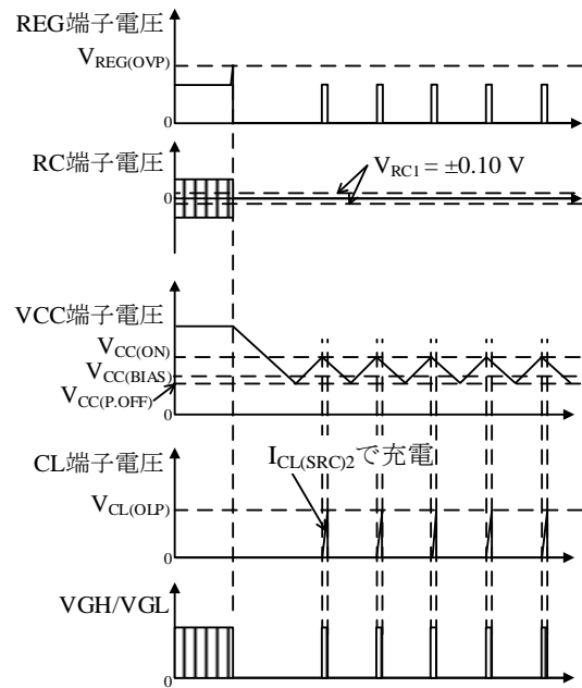
図 8-35 REG_OVP 動作波形
