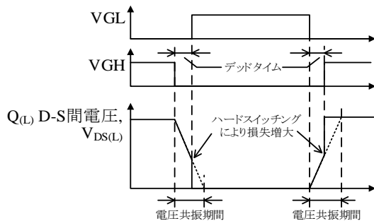
図 8-23 ZVS 不具合波形
