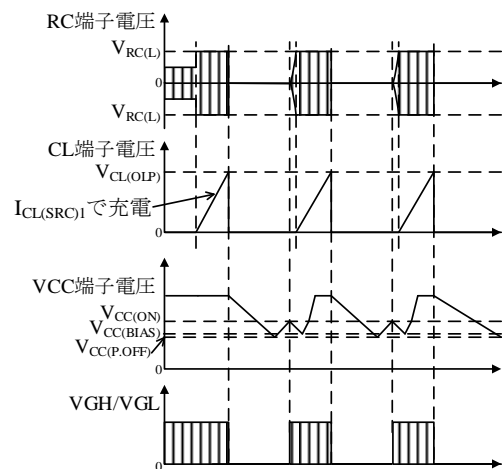
図 8-39 OLP 動作波形
